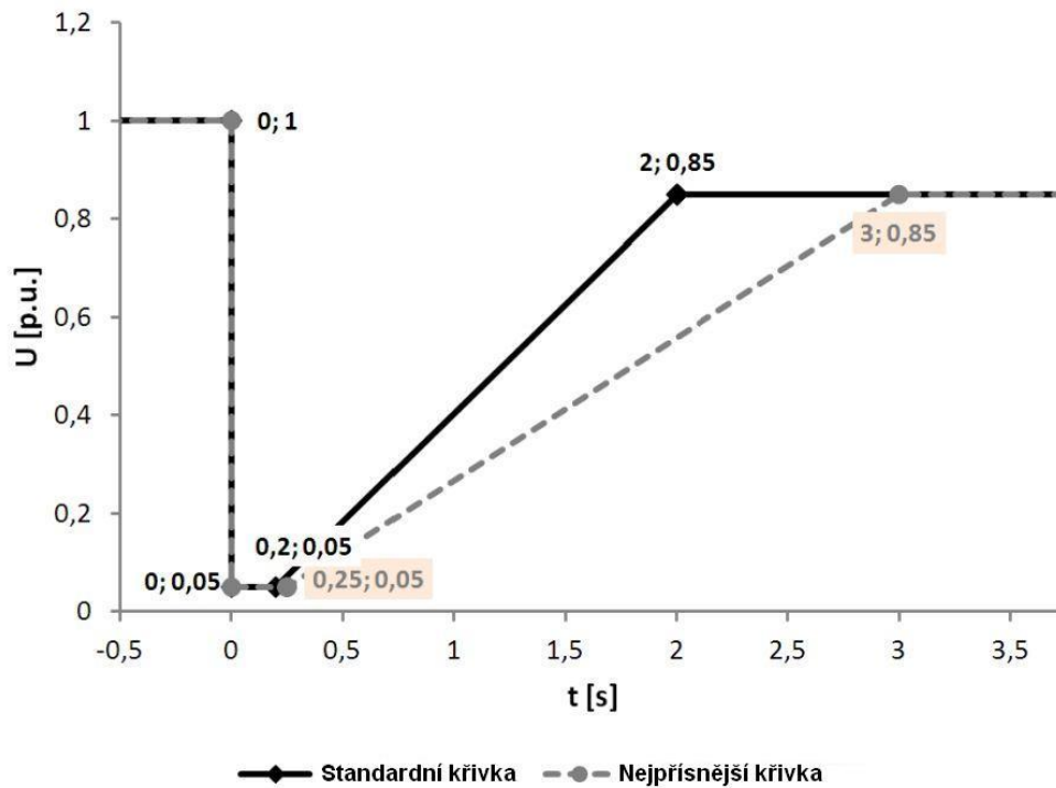
Obr. 7 Schopnost překlenutí poruchy pro výroby se střídačem na výstupu Přímo připojená výrobna
